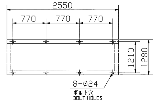
基礎図
