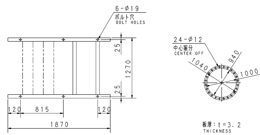
基礎図 FOUNDATION PLAN
