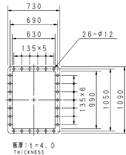
板厚: t=4.0 THICKNESS 吐出しフランジ DISCHARGE FLANGE
