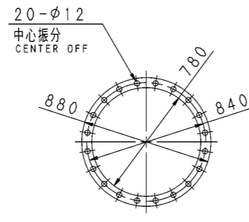
板厚: t=3.2 THICKNESS 吸込フランジ SUCTION FLANGE
