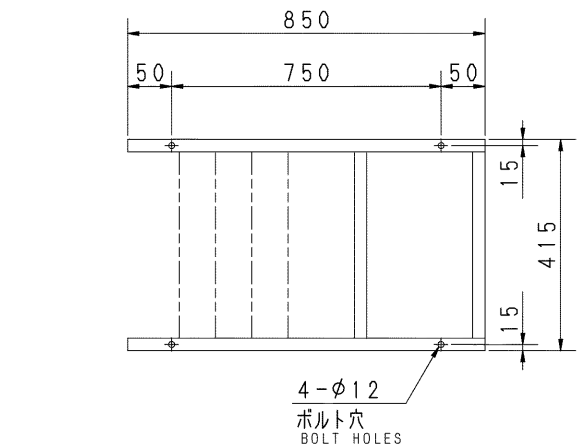
基礎図 FOUNDATION PLAN
