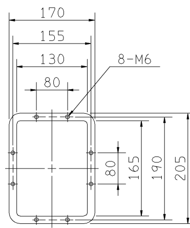
吐出しフランジ DISCHARGE FLANGE
