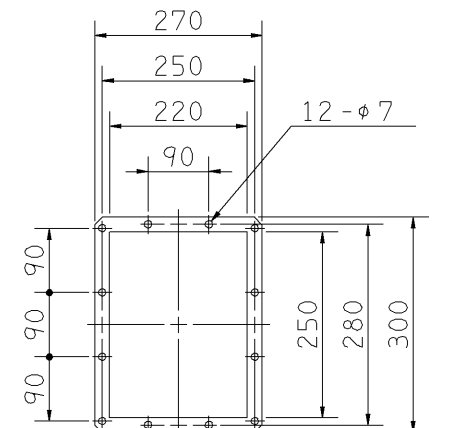
板厚: t=3.0 THICKNESS 吐出しフランジ DISCHARGE FLANGE
