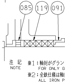
グランドパッキン仕様 (特殊仕様) GLAND PACKINGS SPECIFICATION (OPTION)
