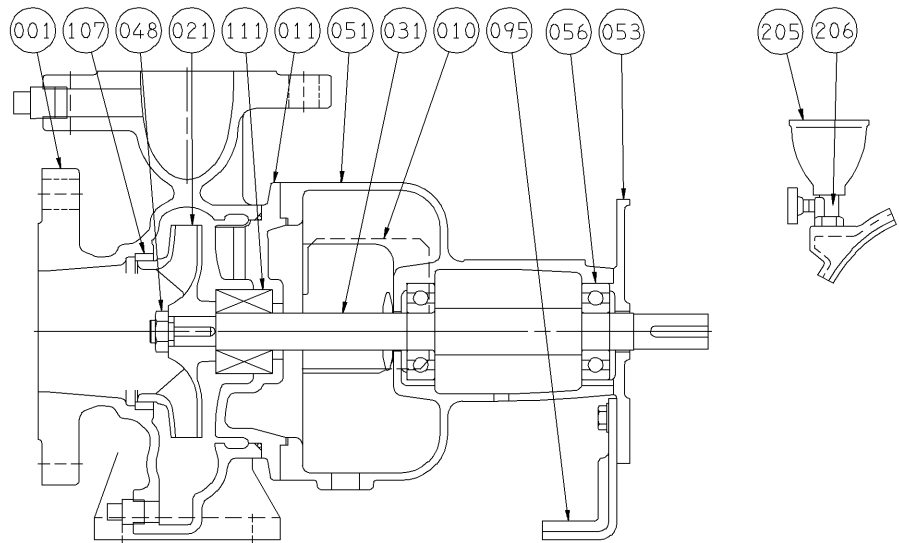
グランドパッキン仕様 (特殊仕様) GLAND PACKINGS SPECIFICATION (OPTION)
