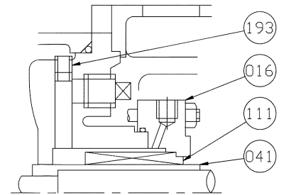
メカニカルシール(特殊仕様) MECHANICAL SEAL(OPTION)
