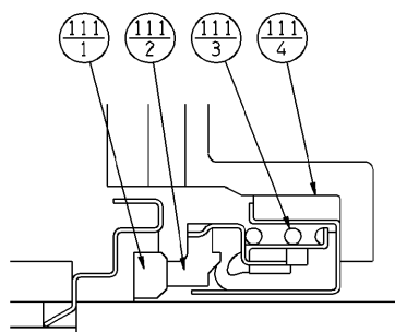
メカニカルシール部詳細 MECHANICAL SEAL
