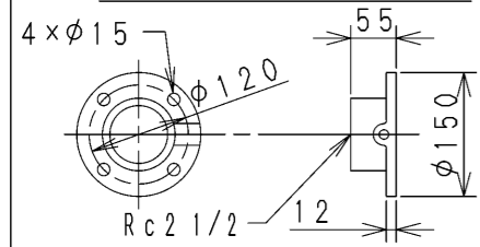
図3 吸込相フランジ 口径: Rc2 1/2
