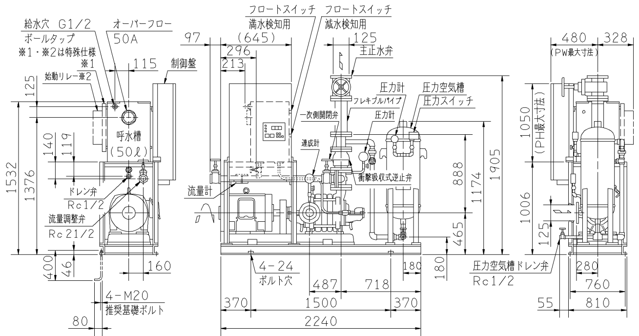
PH, PW寸法減少表 (扉閉空間)
