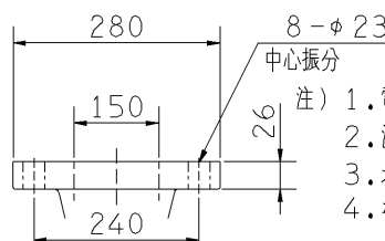
吐出しフランジ
