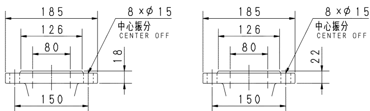
吸込フランジ SUCTION FLANGE
