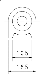
吐出しフランジ DISCHARGE FLANGE
