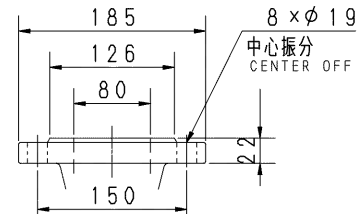
吸込フランジ SUCTION FLANGE
