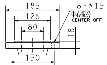
吐出シフランジ DISCHARGE FLANGE
