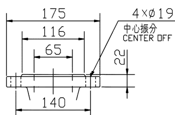
吸水フランジ SUCTION FLANGE
