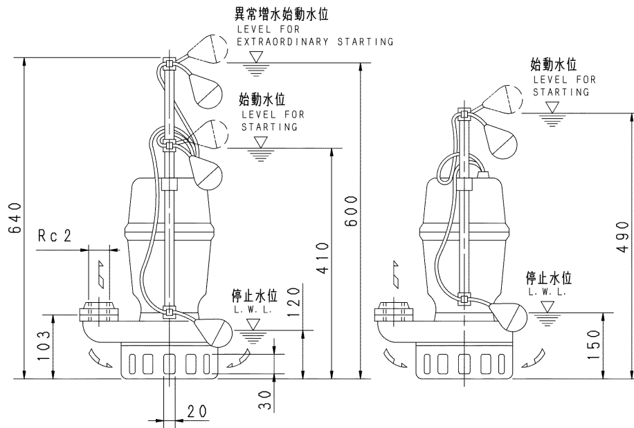
1号機 (DNJ) NO. 1 PUMP
