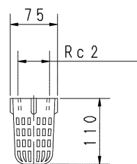
ストレーナ STRAINER
