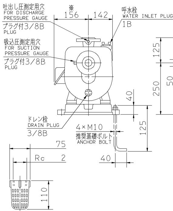
ストレーナ STRAINER
