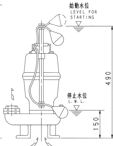
2号機 (DVSA) NO. 2 PUMP
