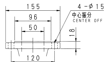
吐出しフランジ DISCHARGE FLANGE
