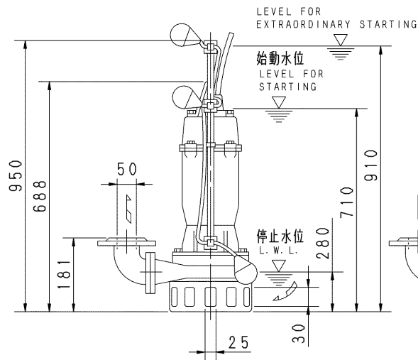
1号機 (DNJ) NO. 1 PUMP
