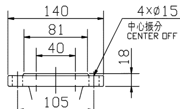
吸込フランジ SUCTION FLANGE
