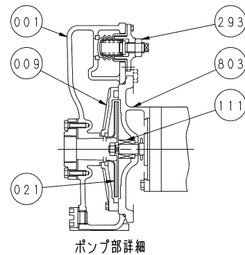
ポンプ部詳細
