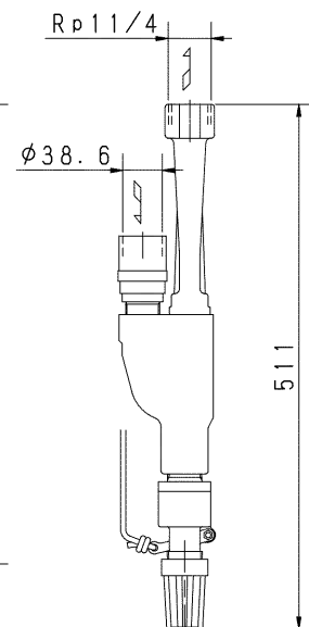
レバー付深井戸ジェット
