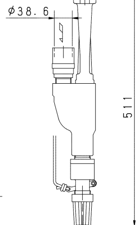
レバー付深井戸ジェット
