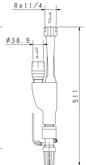
レバー付深井戸ジェット
