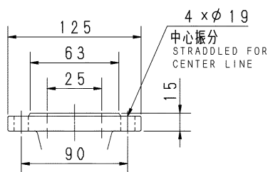
吸引フランジ SUCTION FLANGE
