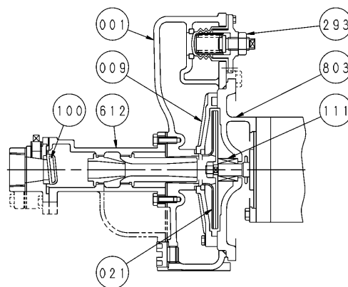
ポンプ部詳細
