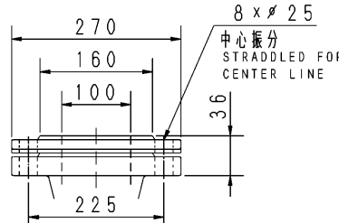
吐出しフランジ DISCHARGE FLANGE
