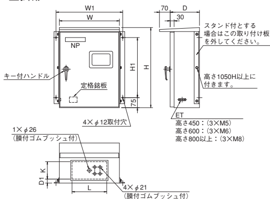
EPC1B型寸法表
