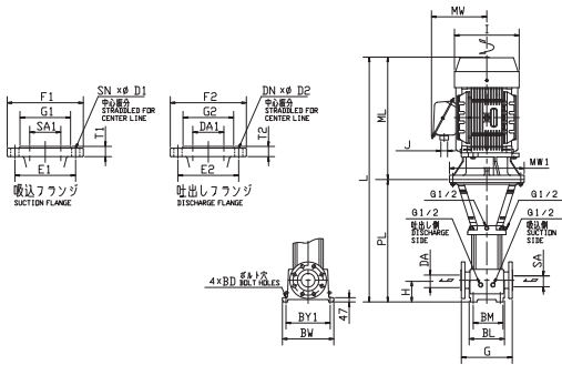
100EVML-R・EVMG-R・EVM-R型
