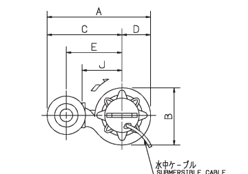
吐出し曲管分割形
