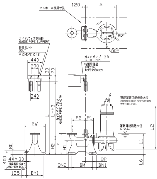
LL型 (LL250, LL300)
