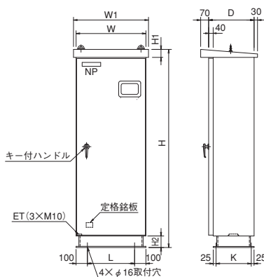
図2 自立形
