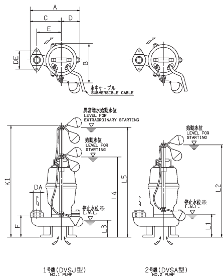
吐出し曲管一体形
