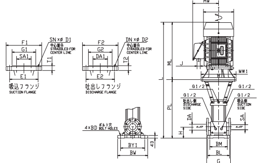
125EVML-R・EVMG-R・EVM-R型
