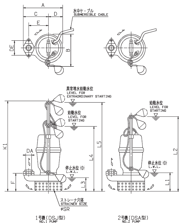
吐出し曲管一体形
