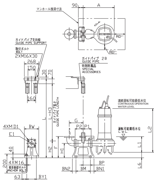
LL型 (LL125, LL150)
