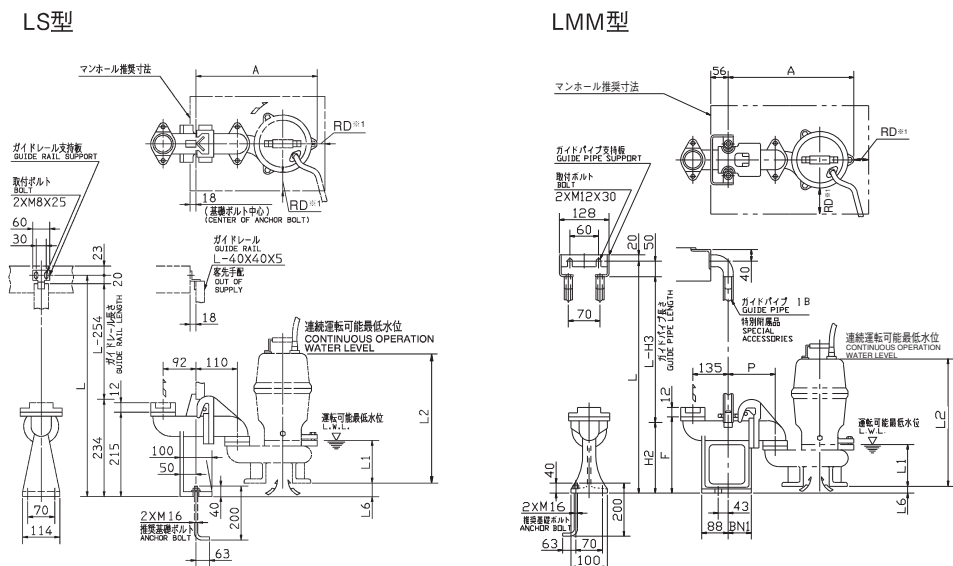
LS型着脱装置付
