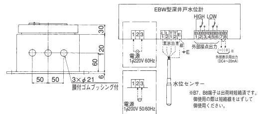
外部結線図
