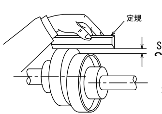
Sをカップリングの周囲4箇所測定し0.05mm以内であれば良好です。 図5: カップリング外周の段違い
