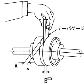
スキメゲージ又はテーパーゲージにてA及びBを上下左右で測定し A及びB : 2~4mm AとBとの差 : 0.1mm以内 であれば良好です。 図6: カップリングの面間誤差
