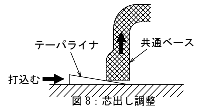
図8: 芯出し調整
