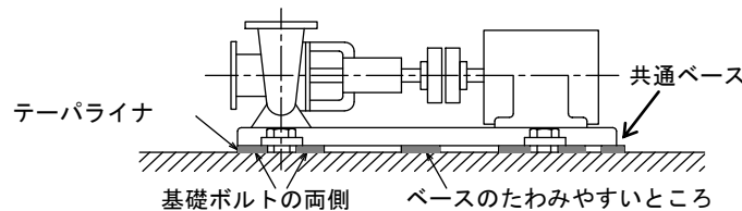
図7: テーパーライナ挿入位置
