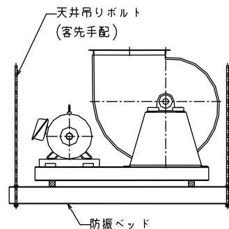
図 6 SRTE3型 (例)
