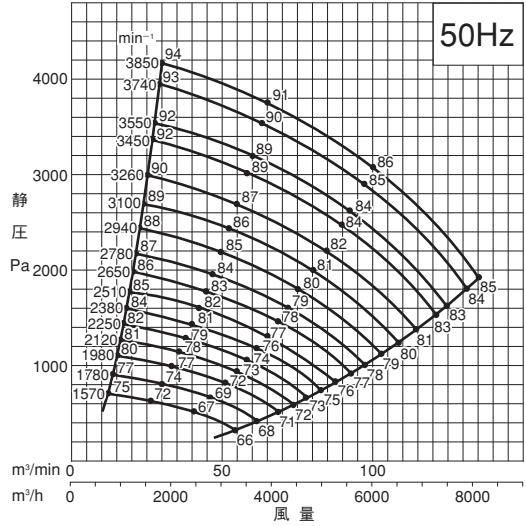
2 1/2 SRPC4型 (4極)
