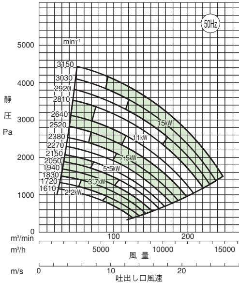
3 SRPC4型 (4極)
