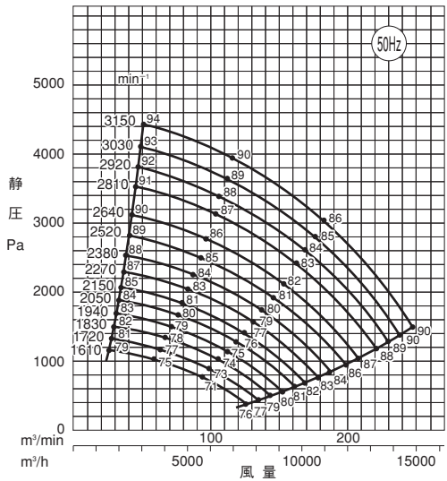
3 SRPC4型 (4極)
