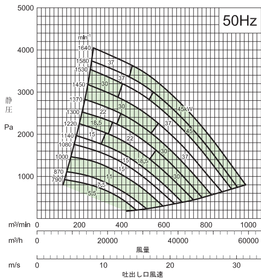
6 SRPC4型 (4極)
