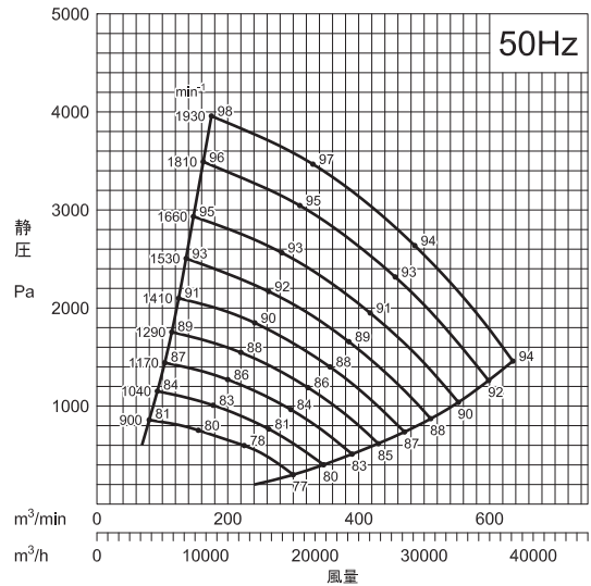
5 SRPC4型 (4極)
