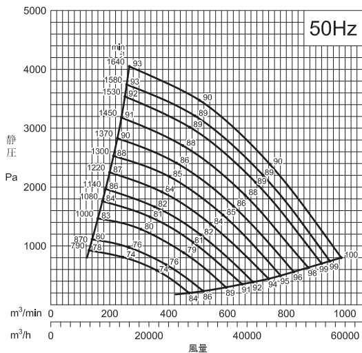
6 SRPC4型 (4極)
