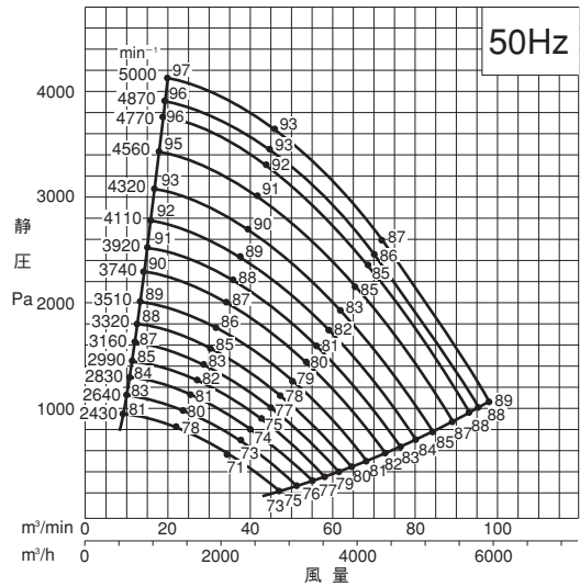
2 SRPC4型 (4極)
