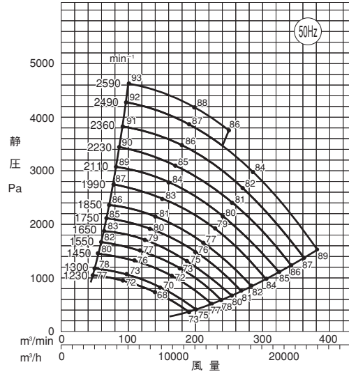
4 SRPC4型 (4極)
