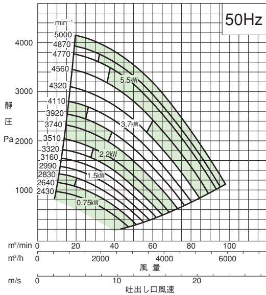
2 SRPC4型 (4極)
