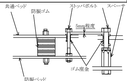
図 5 ストッパボルト取付(例)
