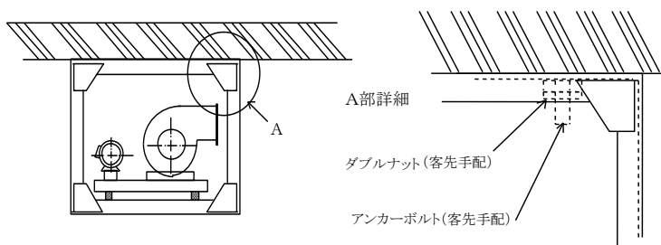
図 7 籠形天井吊り取付(例)
