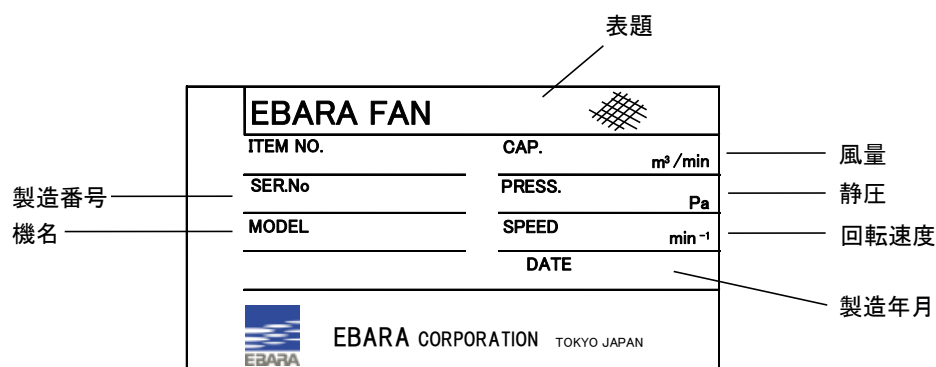
図 1 銘板図
