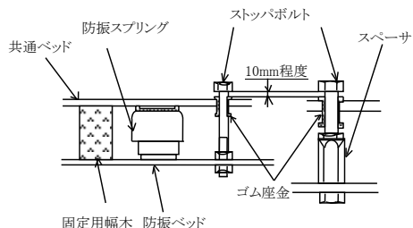
図 6 防振スプリング付の場合
