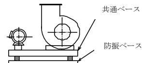
図 2 床置型（例）
