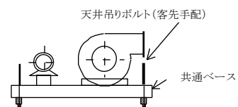
図 4 天井吊り型（例）
