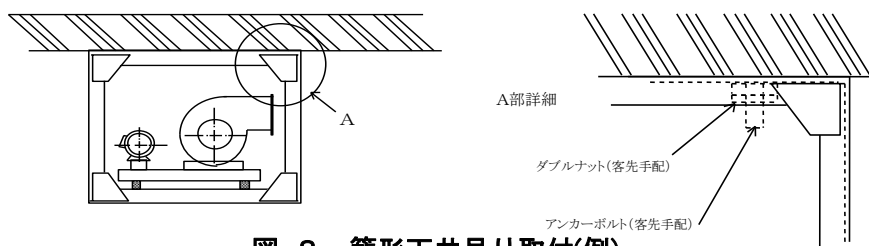
図 8 籠形天井吊り取付(例)
