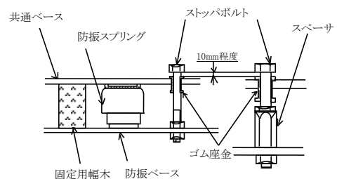
図 7 防振スプリング付の場合
