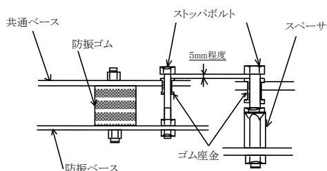
図 6 ストップボルト取付(例)
