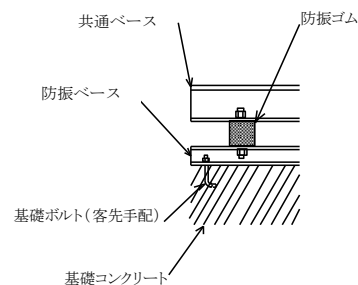
(A) 薄形鋼板防振ベース
