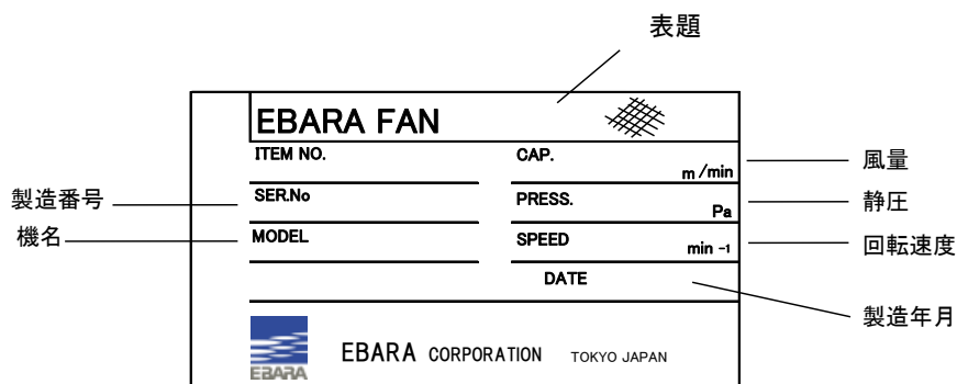
図 1 銘板図
