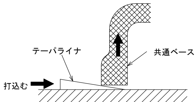
図10 芯出し調整
