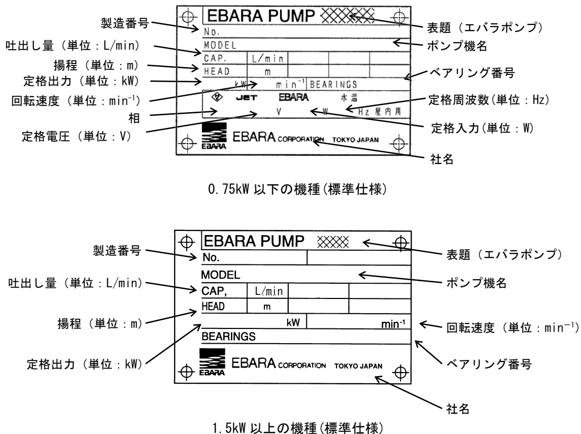
図1 銘板記載事項
