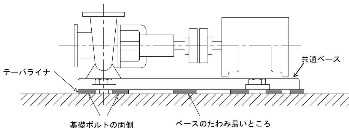
図9 テーパライナ挿入位置
