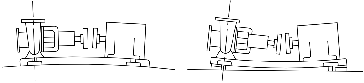
図6 据付時の軸芯のずれ
