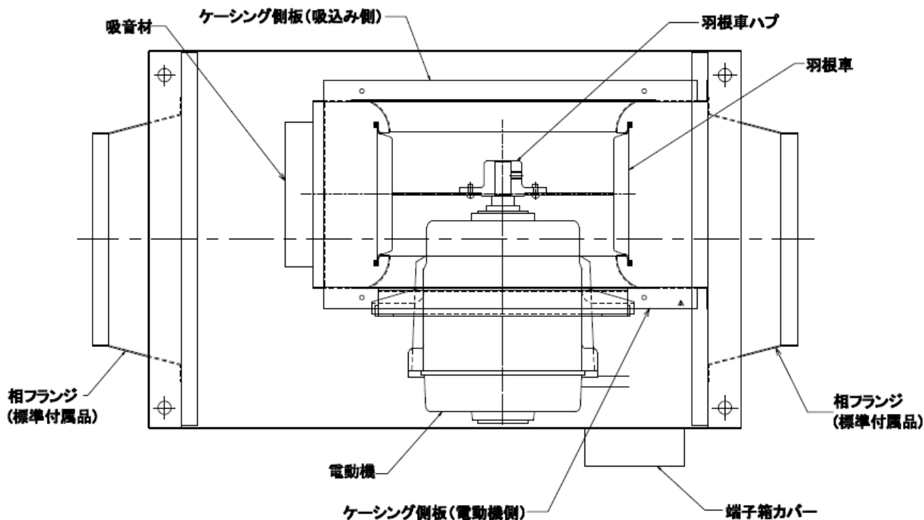
図7 断面図
