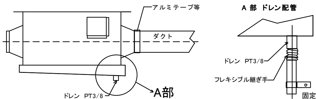
図3 配管方法(吸込側・吐出し側とも)とドレン配管
