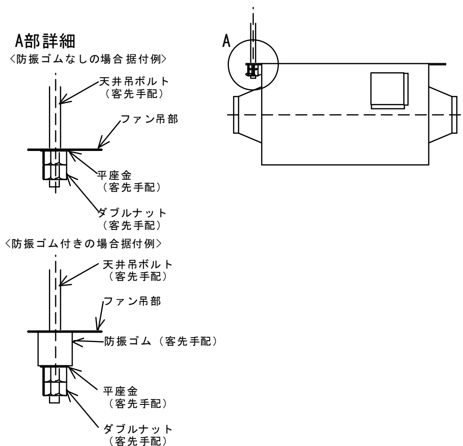
図2 据付方法
