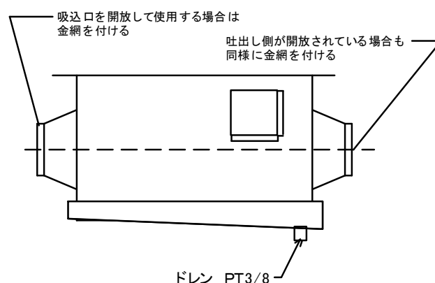
図3 配管方法(吸込側・吐出し側とも)とドレン配管
