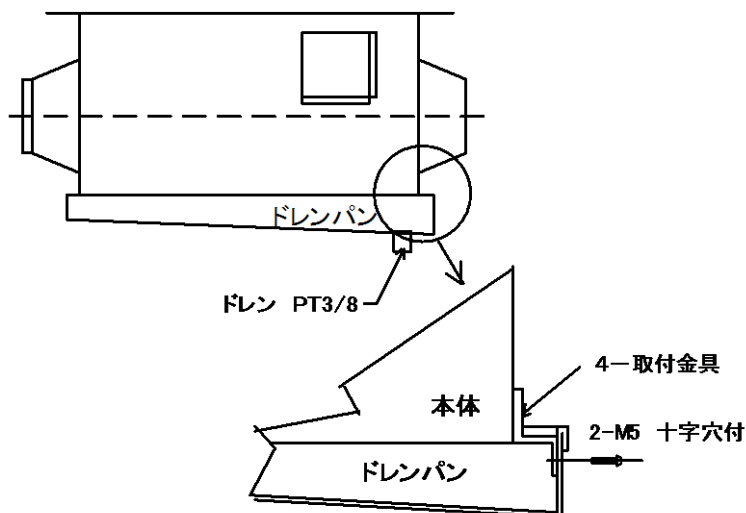
図8 ドレンパン
