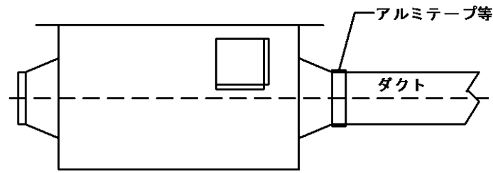
図3 配管方法（吸込側・吐出し側とも）
