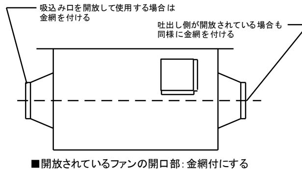
図4 配管上の注意点
