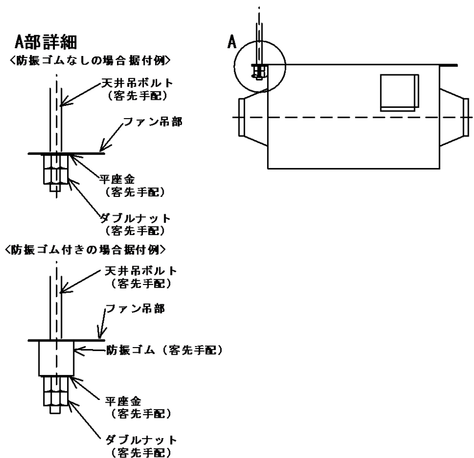
図2 据付方法
