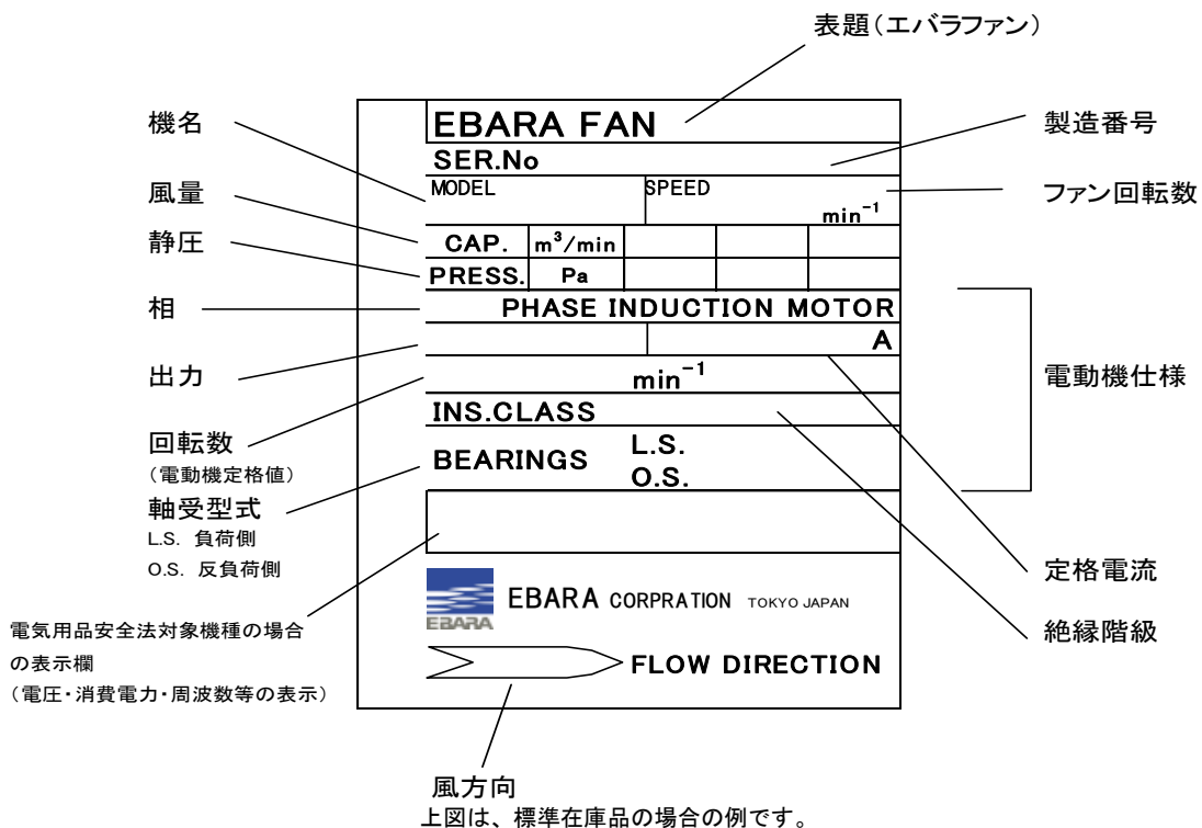
図1 銘板記載事項例
