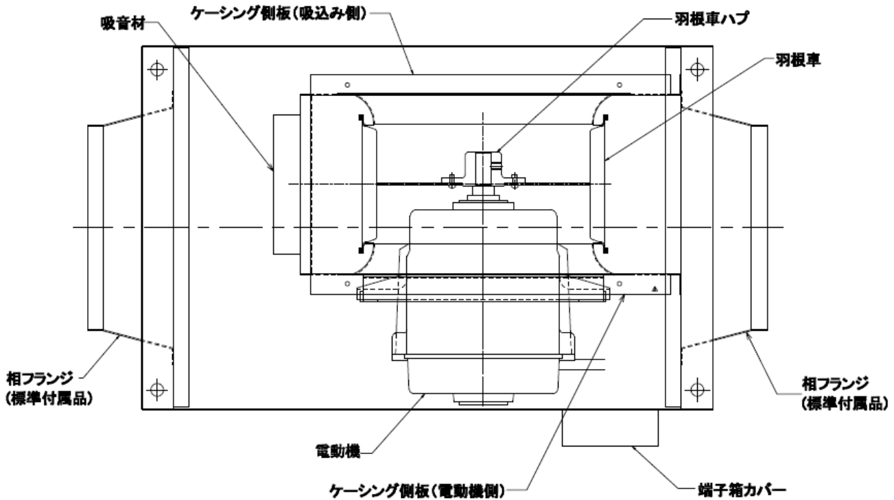
図7 断面図
