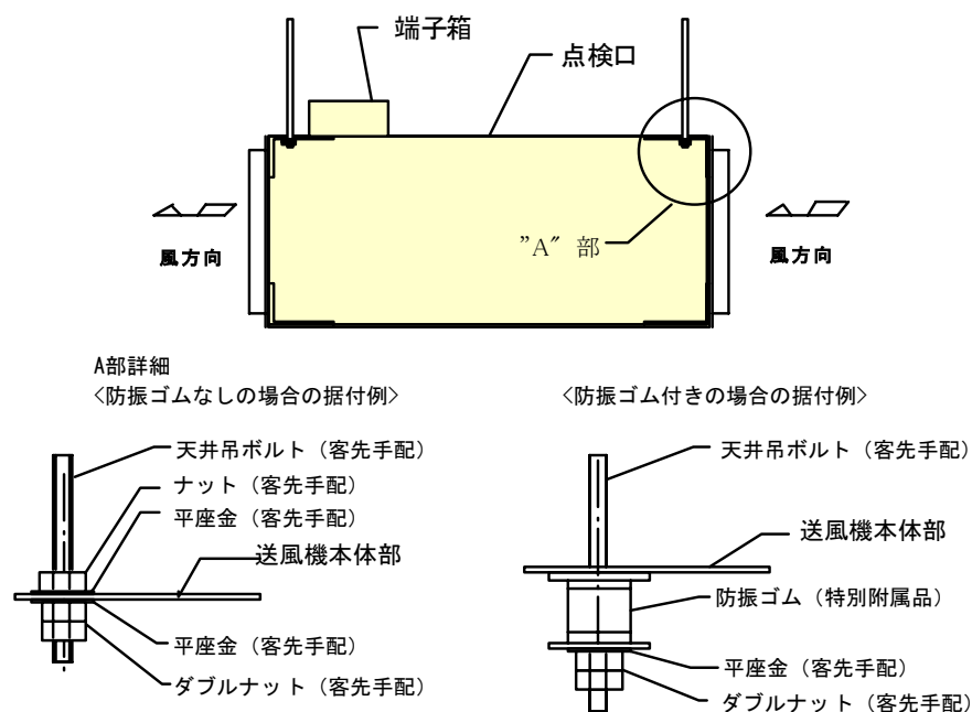
図 2-1 据付方法（天吊り）
