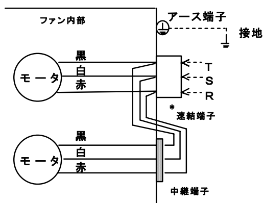
結線図(二台運転型)
