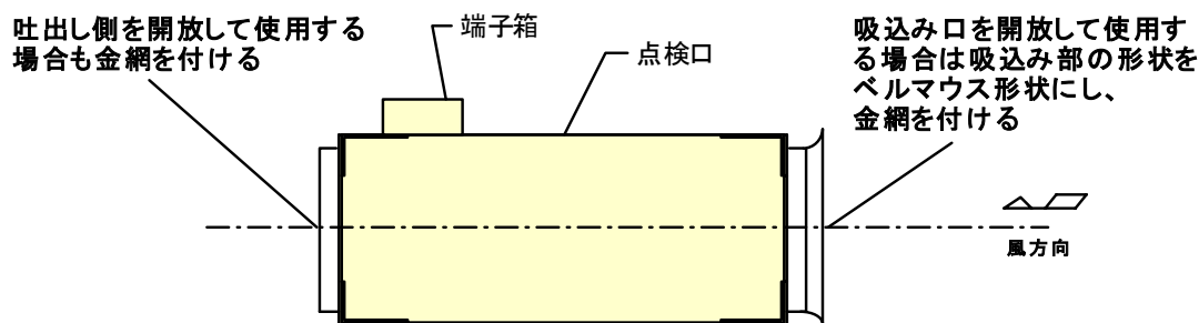
開放されているファンの開口部：金網付にする（客先手配）
