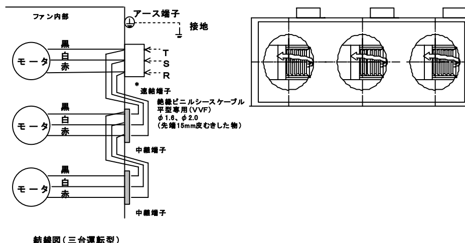
図 5 - 2 結線方法 (三台運転型)
