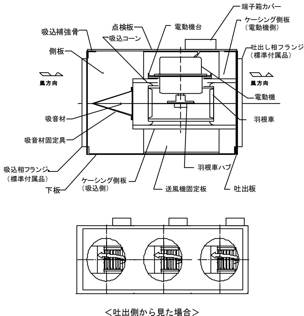
図7 断面図（三台運転型の例）
