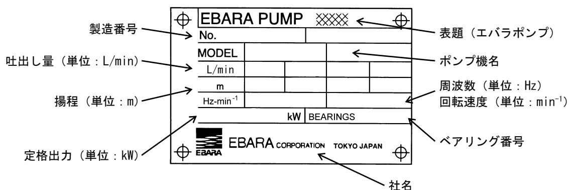
図 1 銘板記載事項 (標準仕様)
