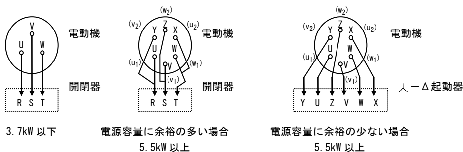
図 2：配線接続図
