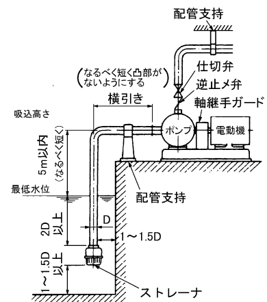
図 2 据付図
