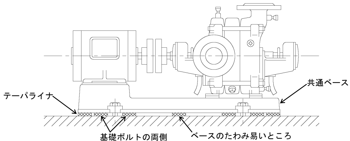
図9 テーパライナ挿入位置
