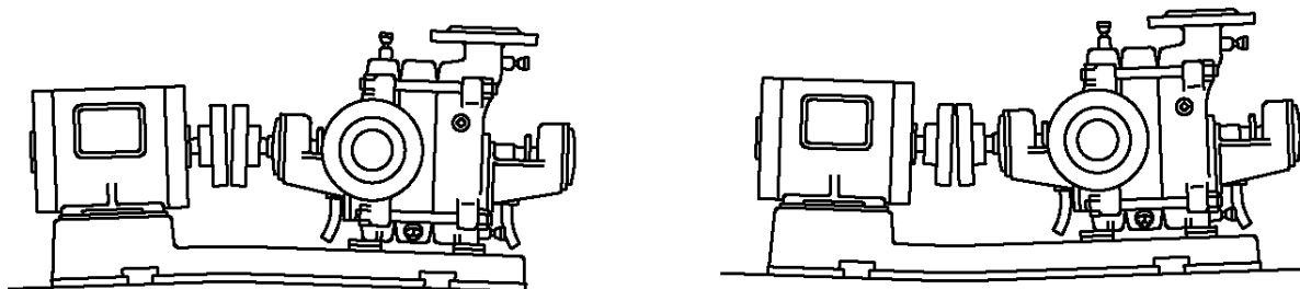
図6 据付時の軸芯のずれ
