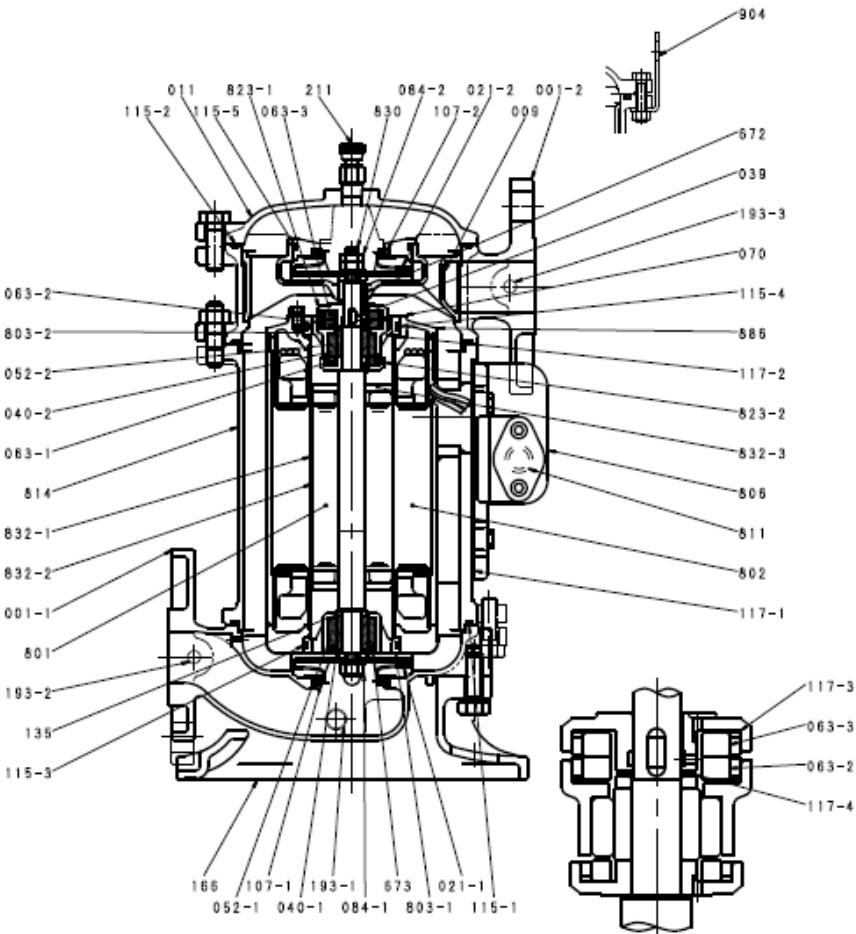
スラスト軸受部詳細
