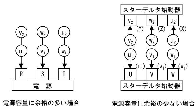
図4 配線接続図
