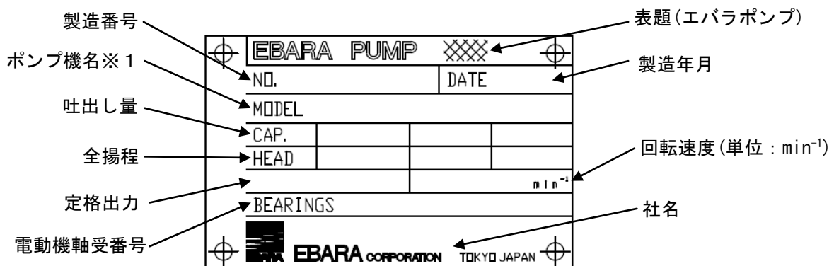
図1 銘板記載事項(標準仕様の場合)
