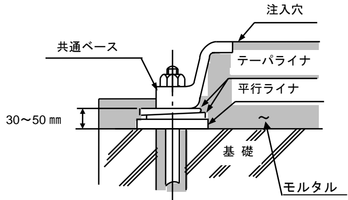
図9：芯出し調整
