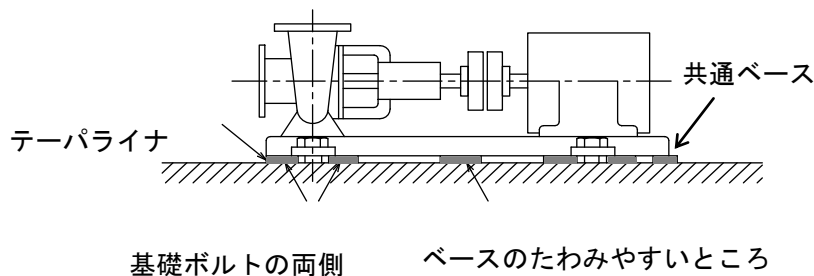
図 8 : テーパーライナ挿入位置
