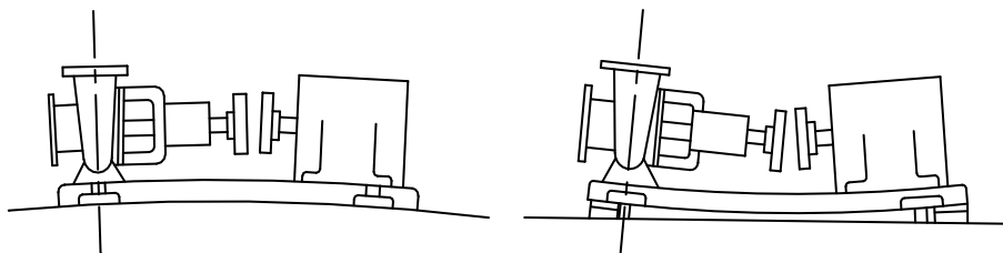
図 5 : 据付時の軸芯のずれ
