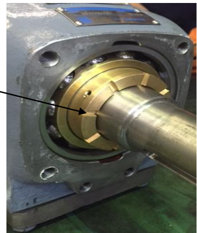
写真 1：油切りリングの溝位置
