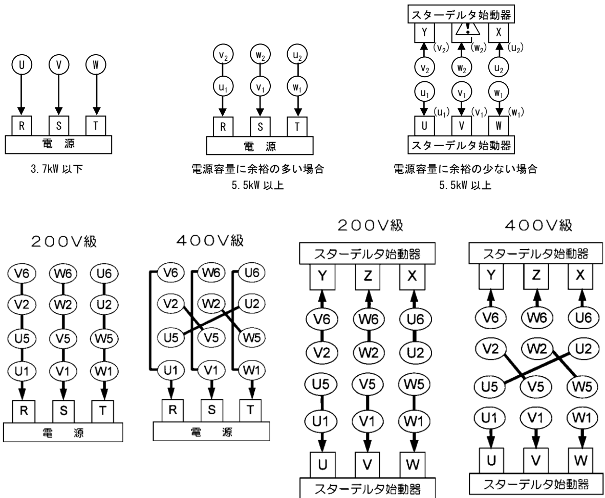
図 10 結線図(代表例)
