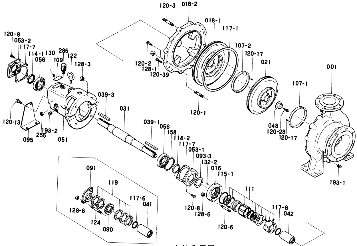
立体分解図
