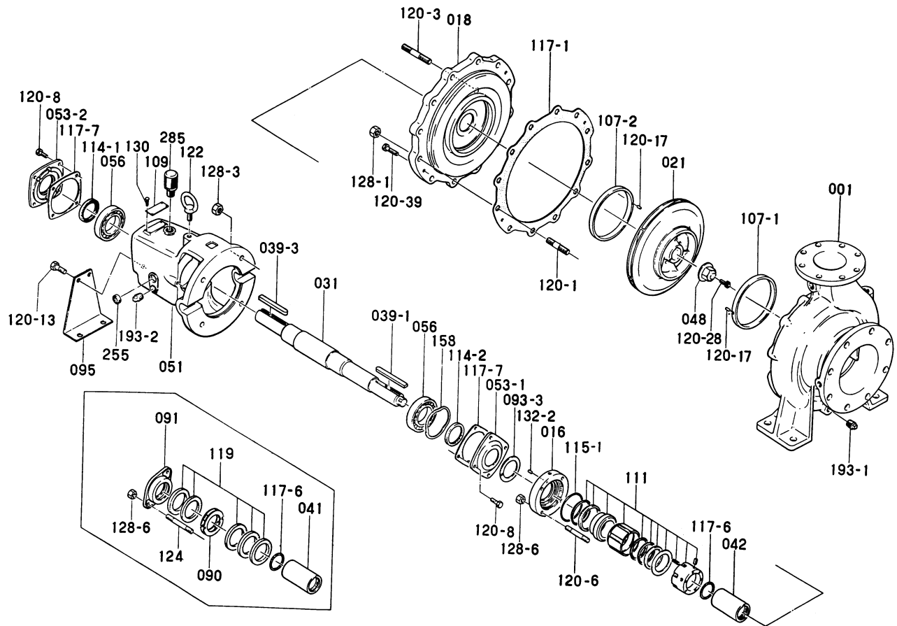
立体分解図
