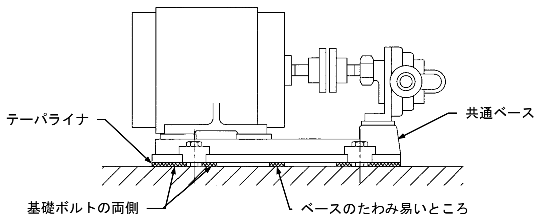
図 10 テーパーライナ挿入位置
