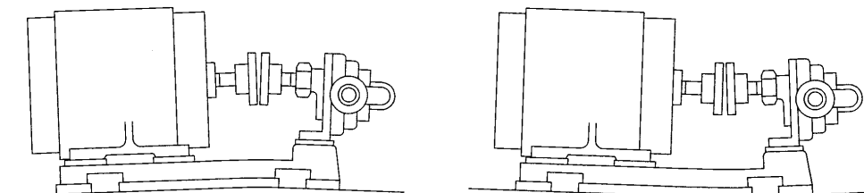
図7 据付時の軸芯のずれ
