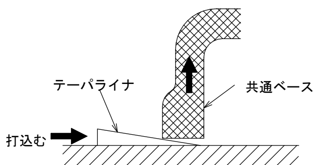
図 11 芯出し調整
