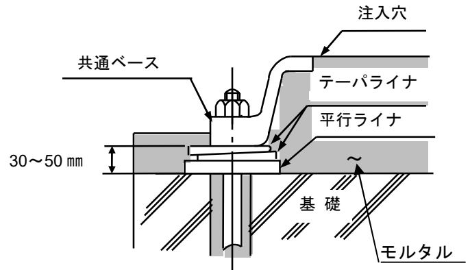
図 7：芯出し調整
