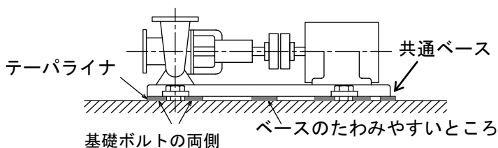
図 8 : テーパライナ挿入位置
