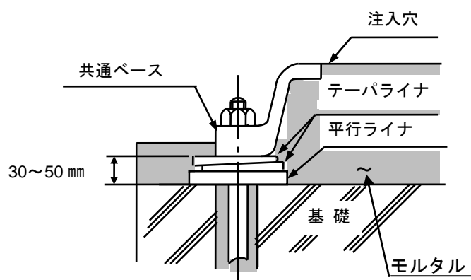
図 9 : 芯出し調整
