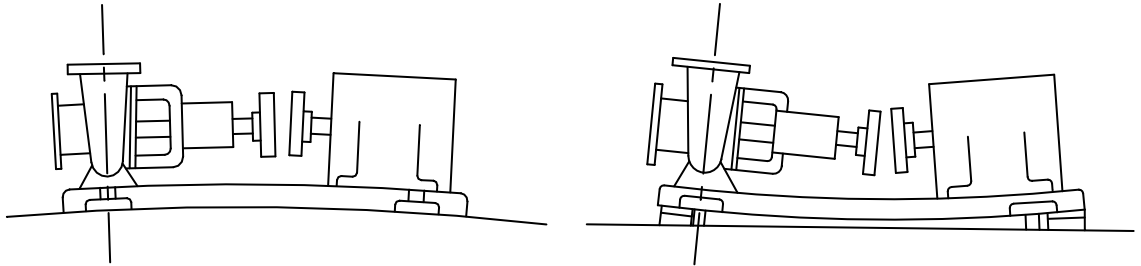
図 5：据付時の軸芯のずれ
